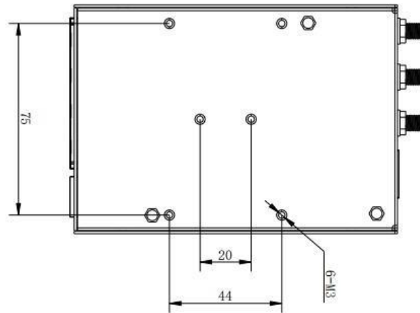
导轨安装位置
